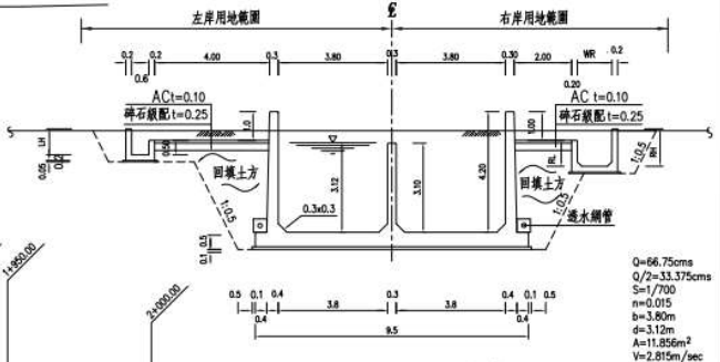
1+600.00~2+100.00 標準断面 比例尺 1:100 單位：M
