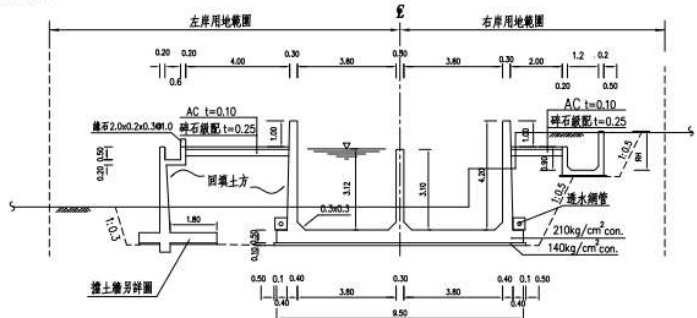
2+100.00~2+300.00 標準斷面
